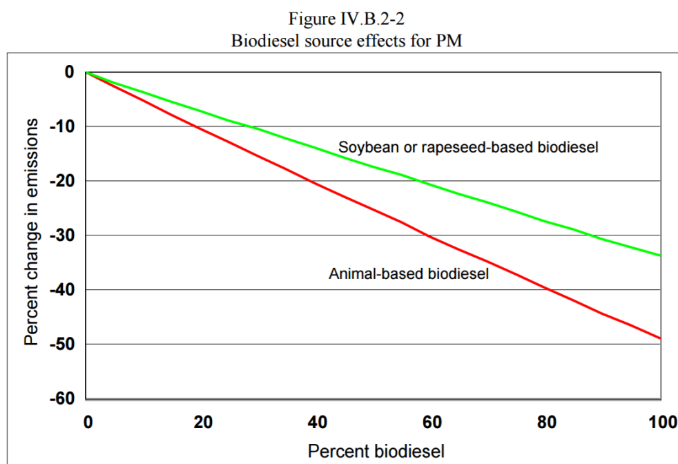
Figura 12 - Relação entre emissão diesel e biodiesel 100
