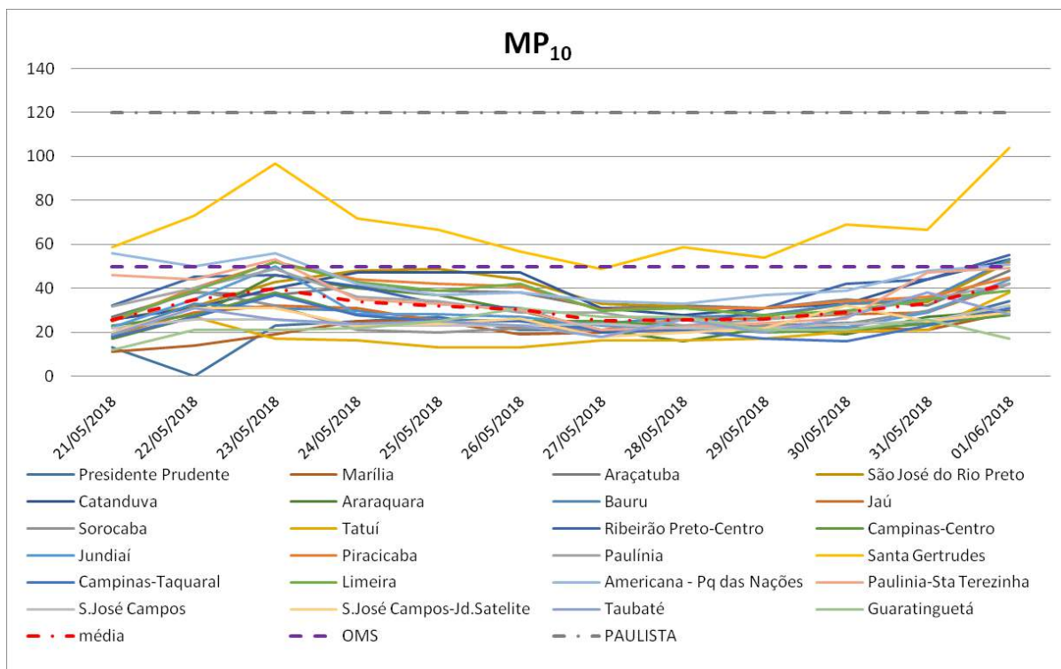
Gráfico 5 – Medidas de concentração de MP10 em 24 estações do interior do estado.
