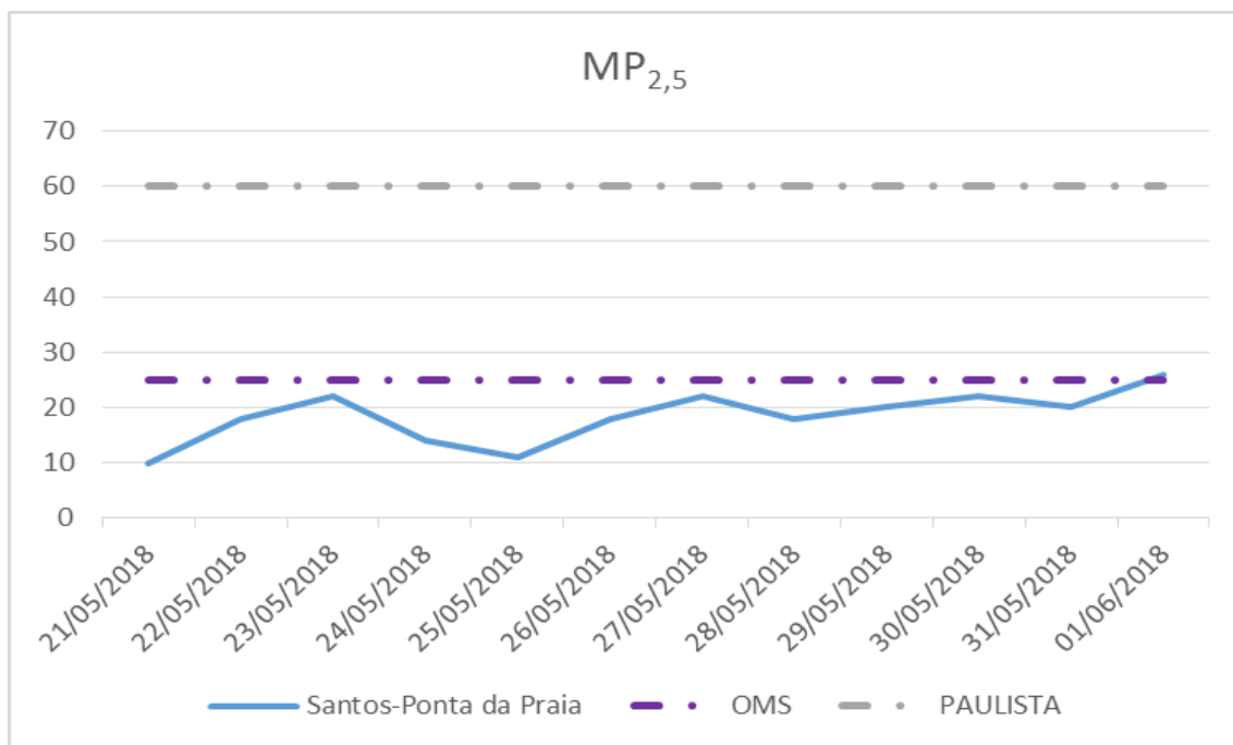
Gráfico 9 – Medida de concentração de MP 2,5 em uma estação em Santos - Baixada Santista.
