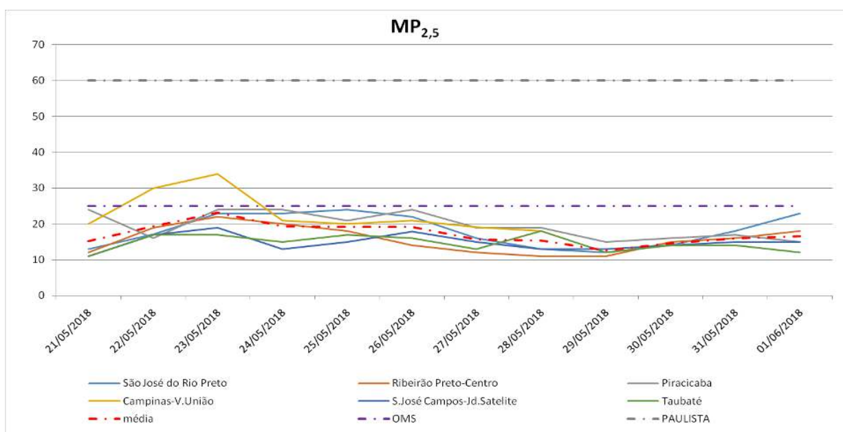
Gráfico 6 – Medidas de concentração de MP_{2,5} em 6 estações do interior do estado.
