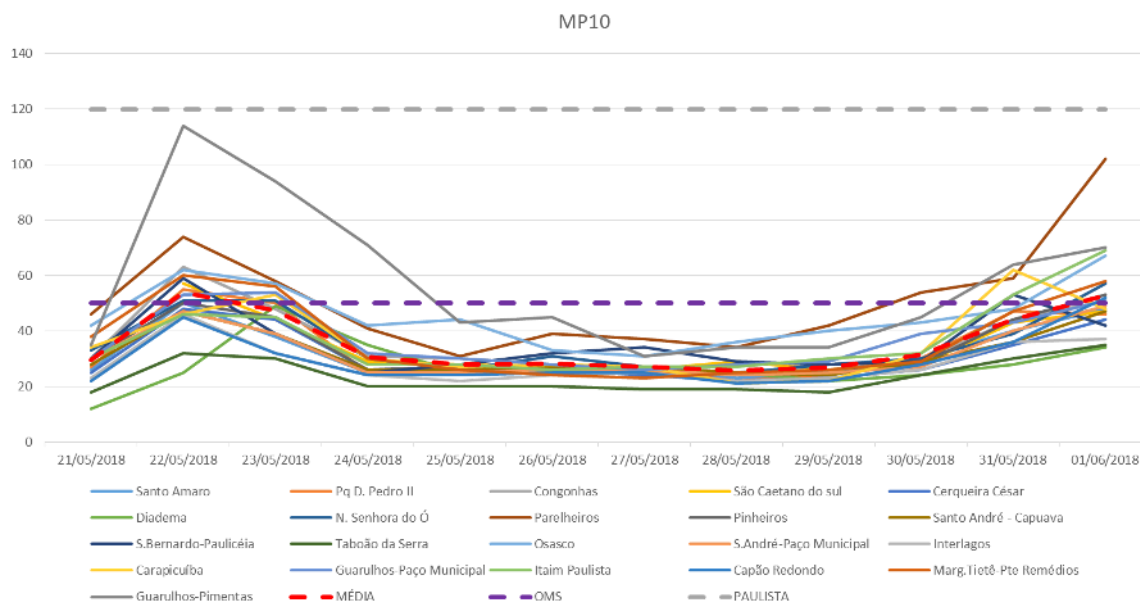
Gráfico 1 – Medidas de concentração de MP10 em 21 estações da RMSP.
